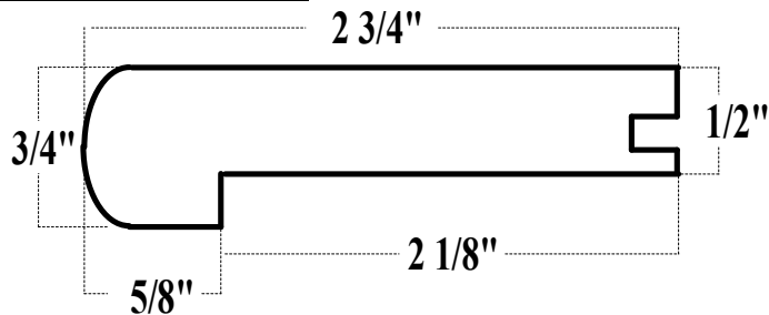
1/2" Flush Stairnose
