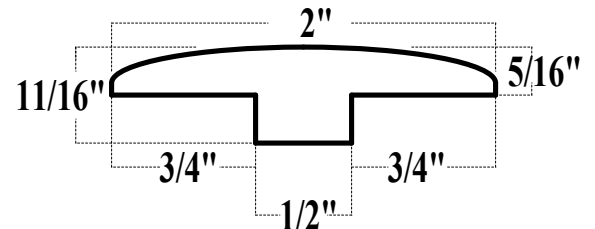
T-Molding
